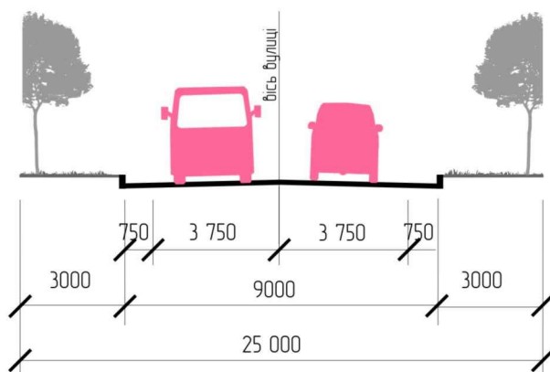
Поперечний профіль Проїзд. М 1:200 (існуючий стан)
