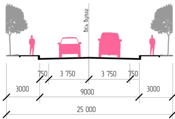
Поперечний профіль Проїзд. М 1:200 (проект)
